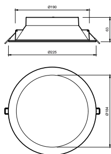
DN029B G2 LED20 3CCT 24W D200 DIM AU
