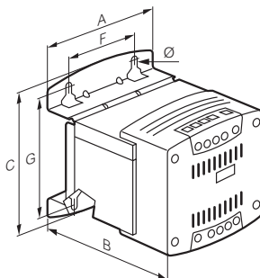
Fig. 4: 4000 to 8000 VA
