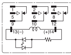
3PDT
