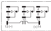
3PDT
