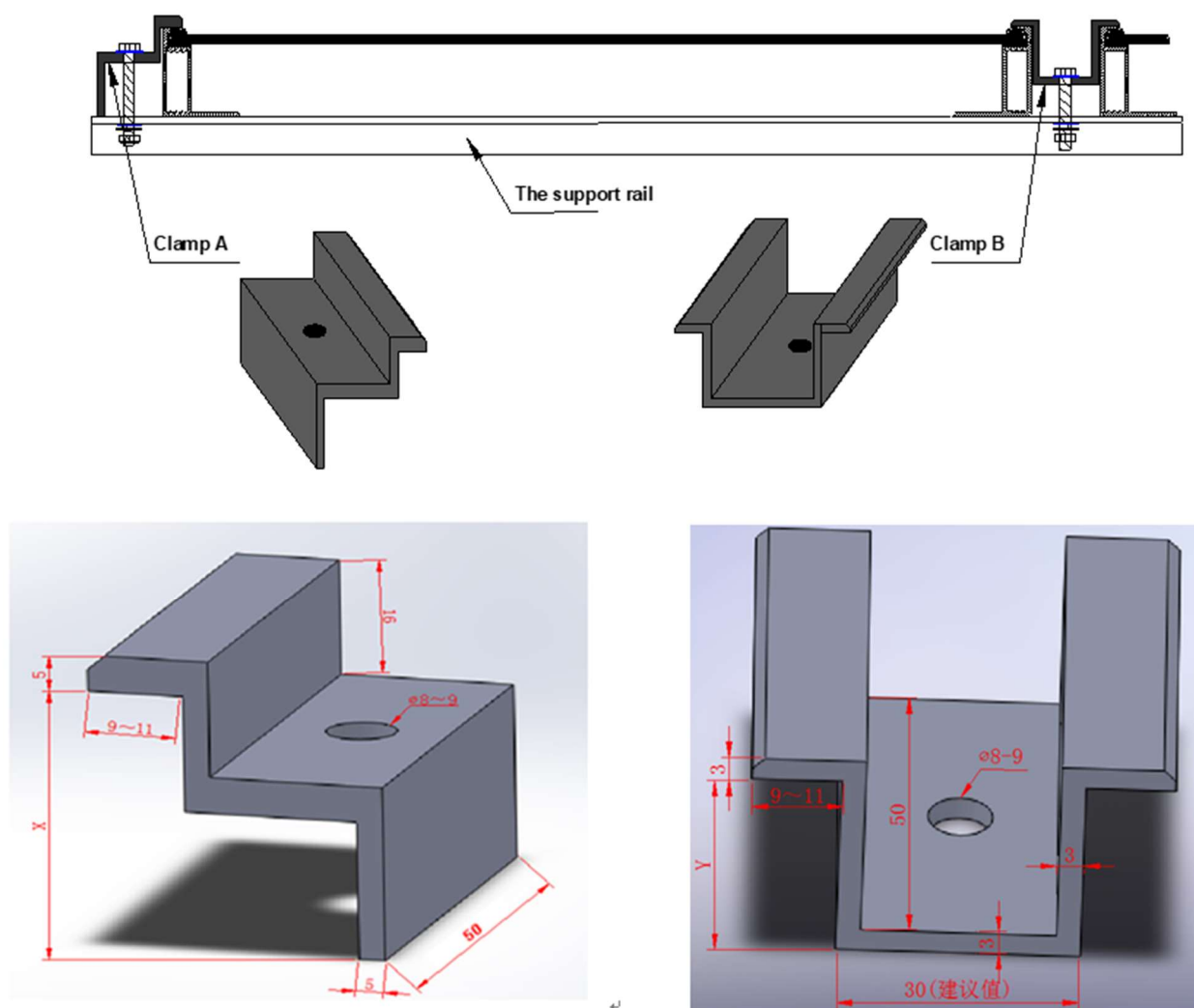
Fixture A: Fixture for edge module
